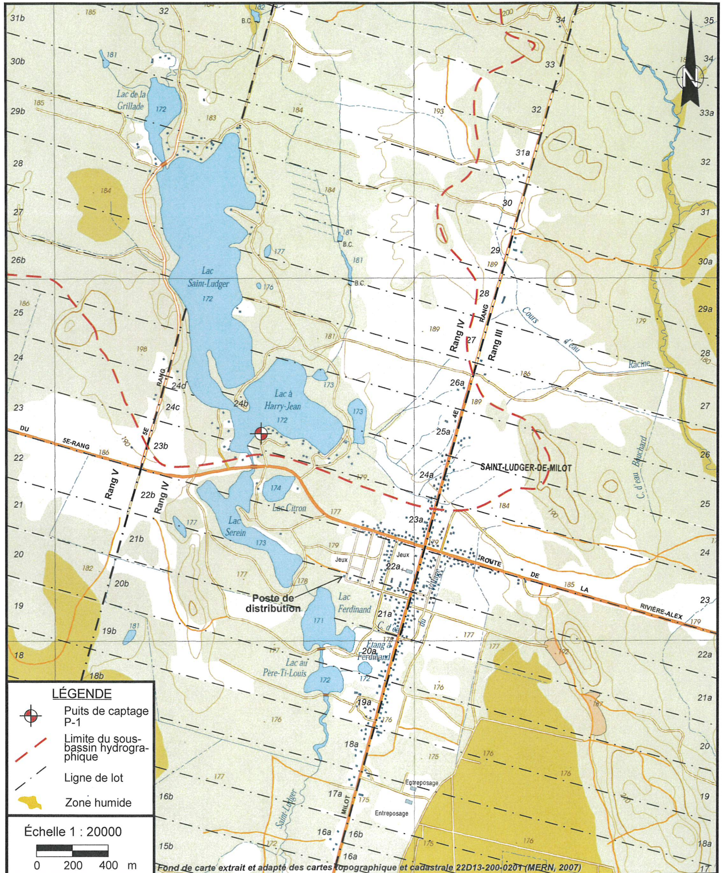
Figure 1. Localisation du puits de captage P-1 sur le territoire municipal de Saint-Ludger-de-Milot
