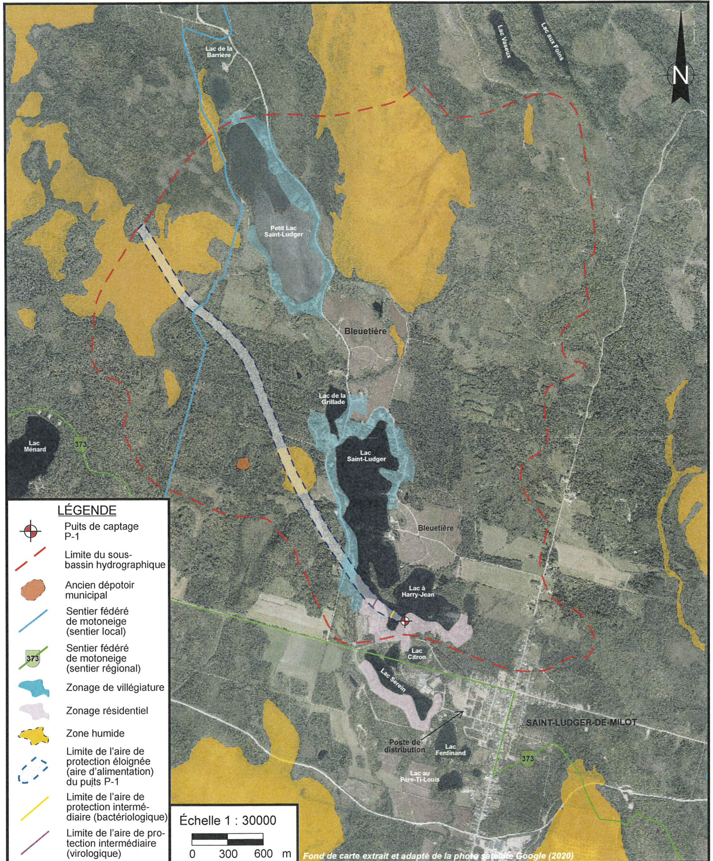
Figure 5. Configuration de l'aire de protection éloignée du puits de captage P-1 de Saint-Ludger-de-Milot
