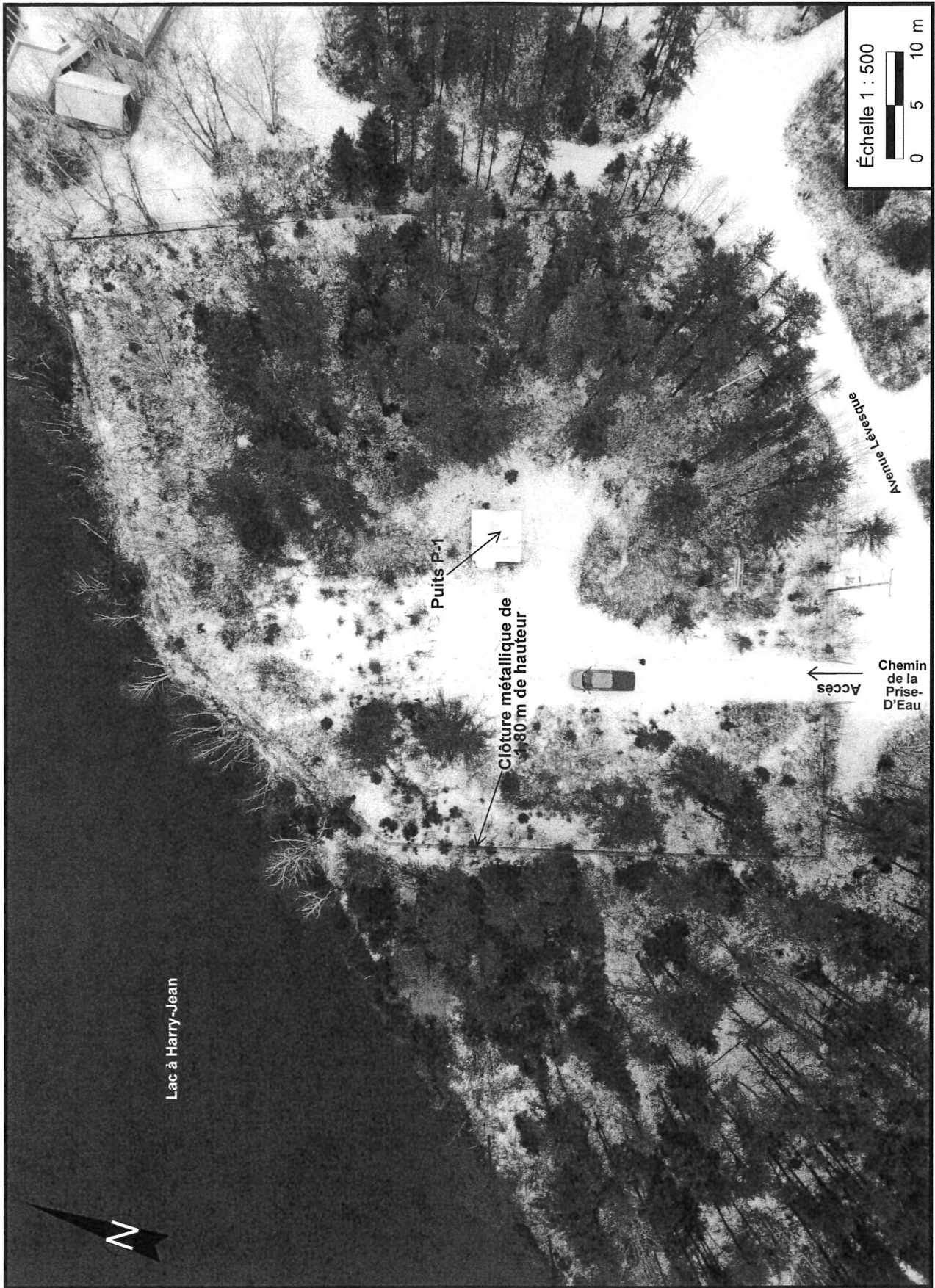
Figure 3. Configuration de l'aire de protection immédiate autour du puits de captage P-1 (photo aérienne prise le 18 nov. 2020)
